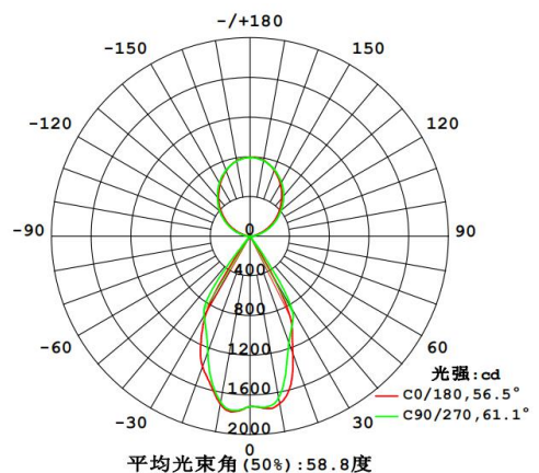
格栅 60°
