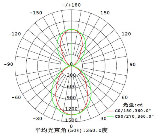
棱镜面罩
