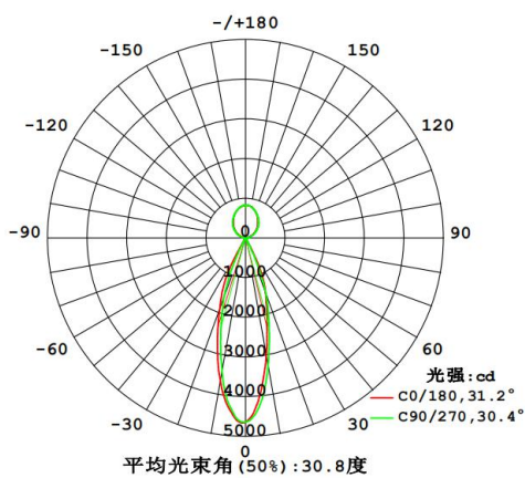
格栅 30°
